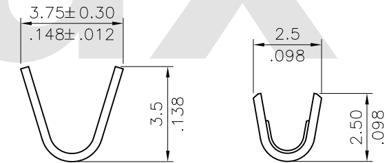
SEC:A-A
