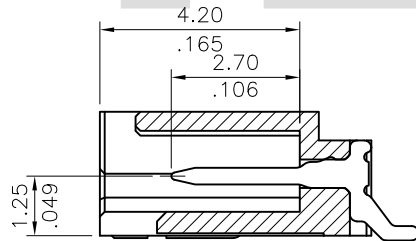
SEC. A-A
