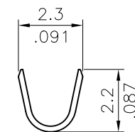
SEC.: A-A
