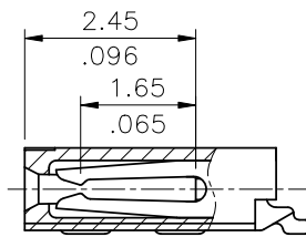
SEC.:Y-Y
