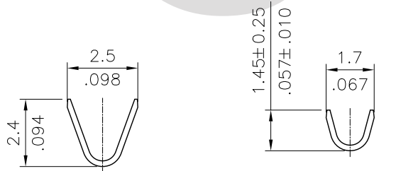
SEC.: A-A
