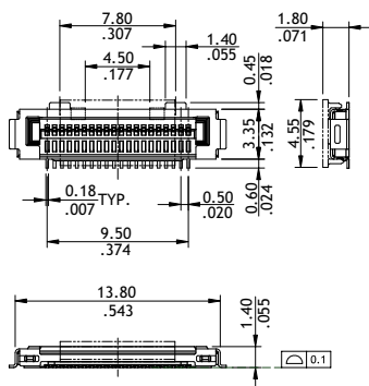
P/N CVS320*M1R0-NH
