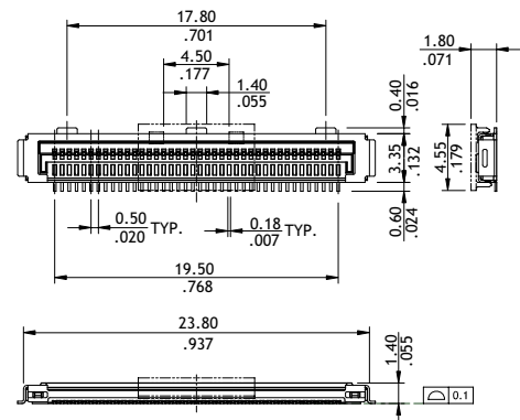
P/N CVS340*M1R0-NH
