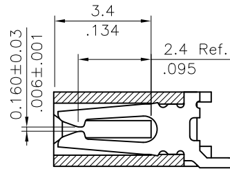
A-A SEC.
