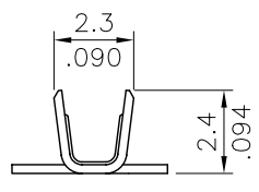
SEC.: A-A P/N:CI94TM3*PPO
